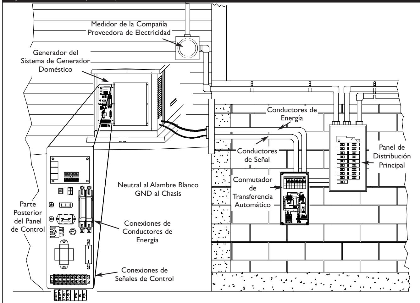
Figura 7 — Instalación Típica Completa del Conmutador de Transferencia Automático
